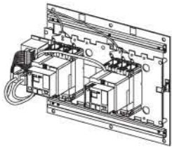
ATS NSX100-630
